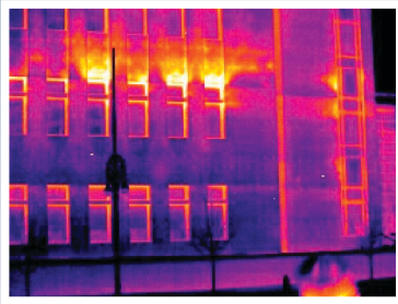
Air Exfiltration
