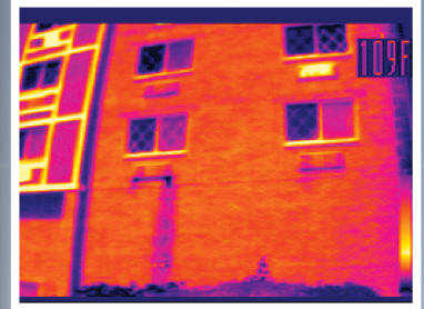
Moisture Intrusion
